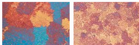
Δομή χυτού Heraenium CE χωρίς κερί KF (αριστερά) και με κερί KF (δεξιά)
