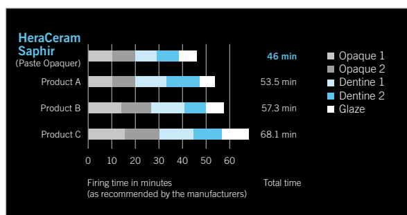
Εικ. 2 Εξαιρετικά σύντομοι χρόνοι όπτησης.
