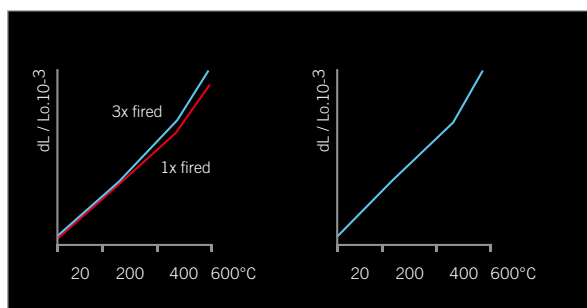
Εικ. 3 Σύγκριση αύξησης CTE. Ασταθές CTE άλλου οδοντιατρικού κεραμικού μετά από πολλαπλές οπτήσεις
