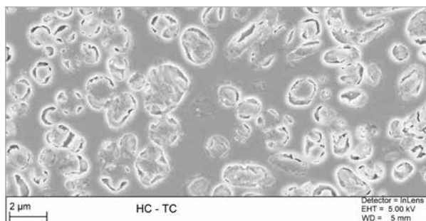
Εικ. 1 HeraCeram μικρογραφία αδροποίησης με τη δομή λευκίτη.
